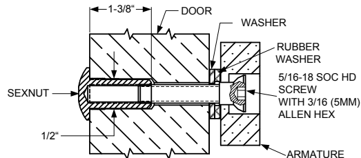
FIG. 2B SOLID DOOR
